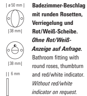
Badezimmerbeschlag-satz mit runden Rosetten, Verriegelung und Rot/Weiß-Scheibe. Ohne Rot/Weiß-Anzeige auf Anfrage. Bathroomfitting, round roses, thumbturn and red/white indicator. Without red/white indicator on request.
